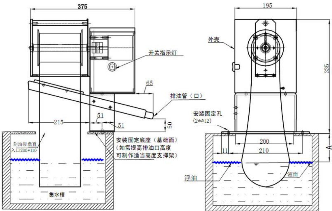
图1：产品规格及安装示意图
