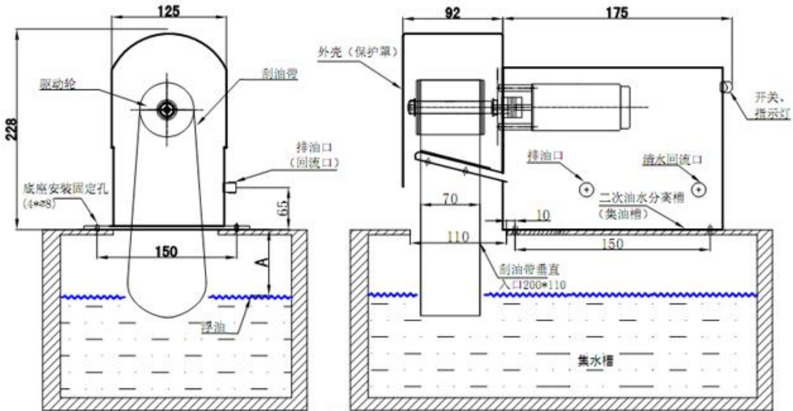
安装、工作原理示意图 注：如订货请提供“A”尺寸，以便配置刮油带长度！
